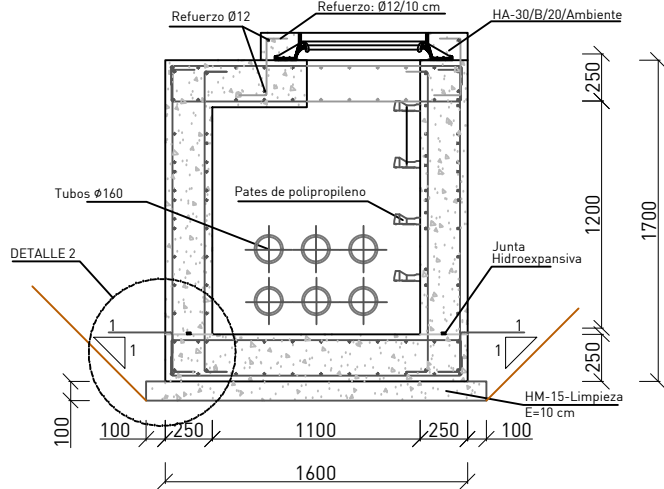
Sección B-B'
